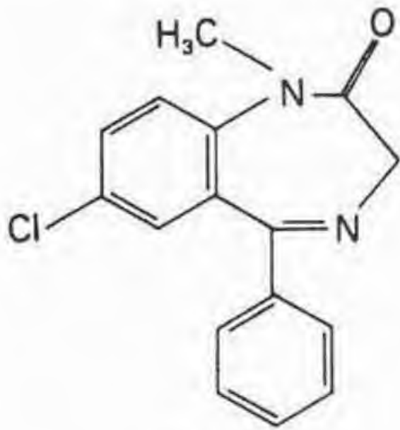
VALIUM
